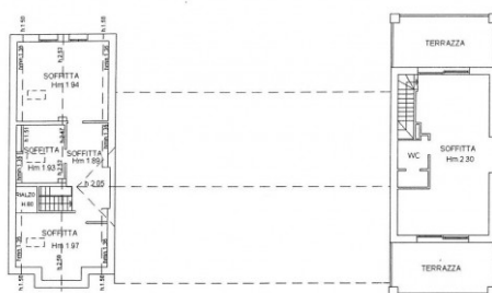
PIANO PRIMO
