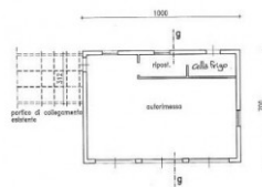
pianta piano terra - scala 1:100
